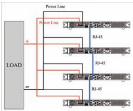
Configuración Paralela
